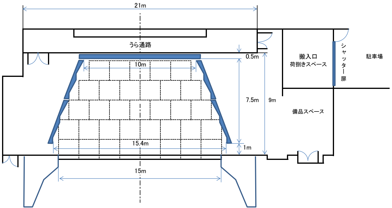
舞台平面図 反射板＋平台配置図
