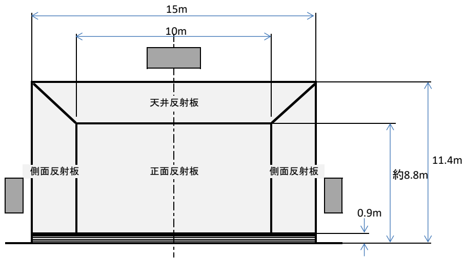
舞台正面図 反射板＋平台配置図
