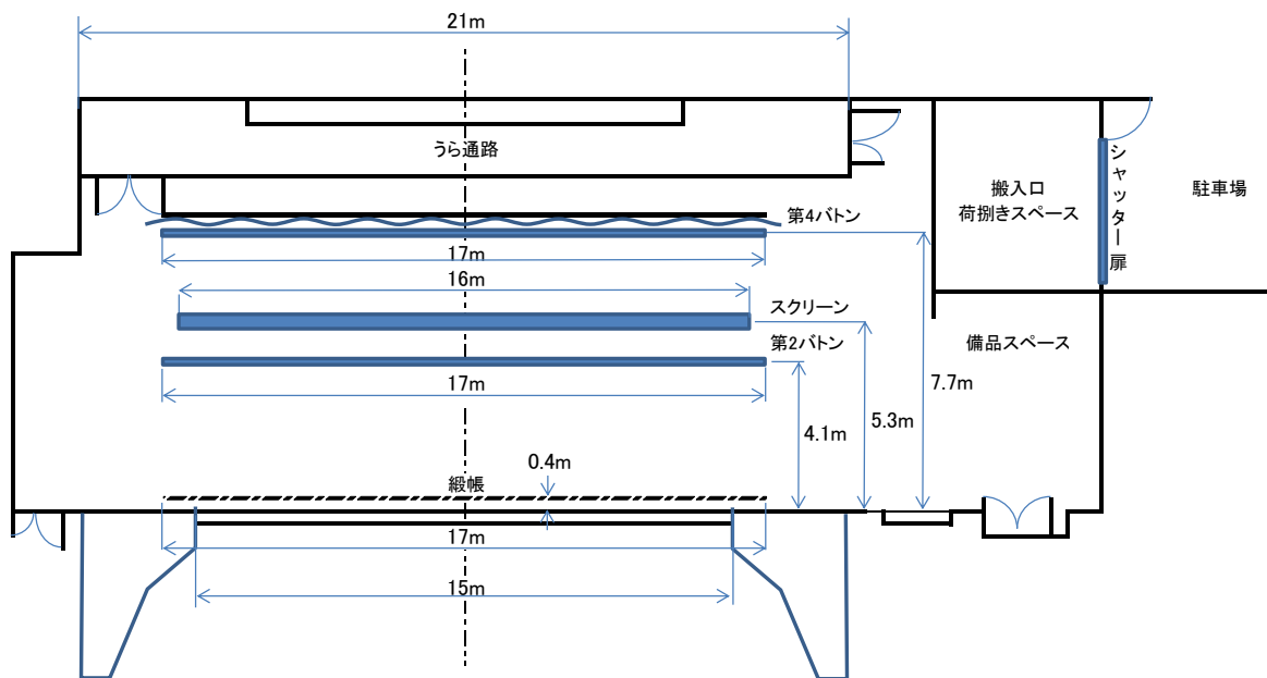
舞台平面図 スクリーン・パトン配置図
