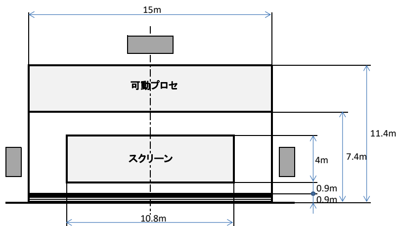
舞台正面図 スクリーン・パトン配置図
