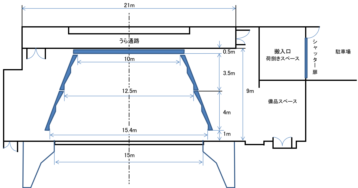
舞台平面図 反射板配置図
