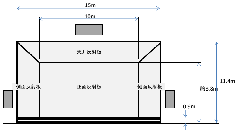
舞台正面図 反射板配置図
