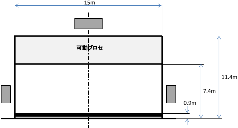
舞台正面図 空舞台
