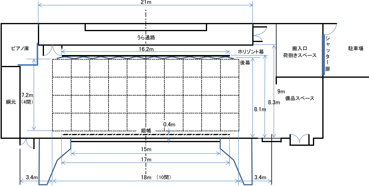
舞台平面図 空舞台
